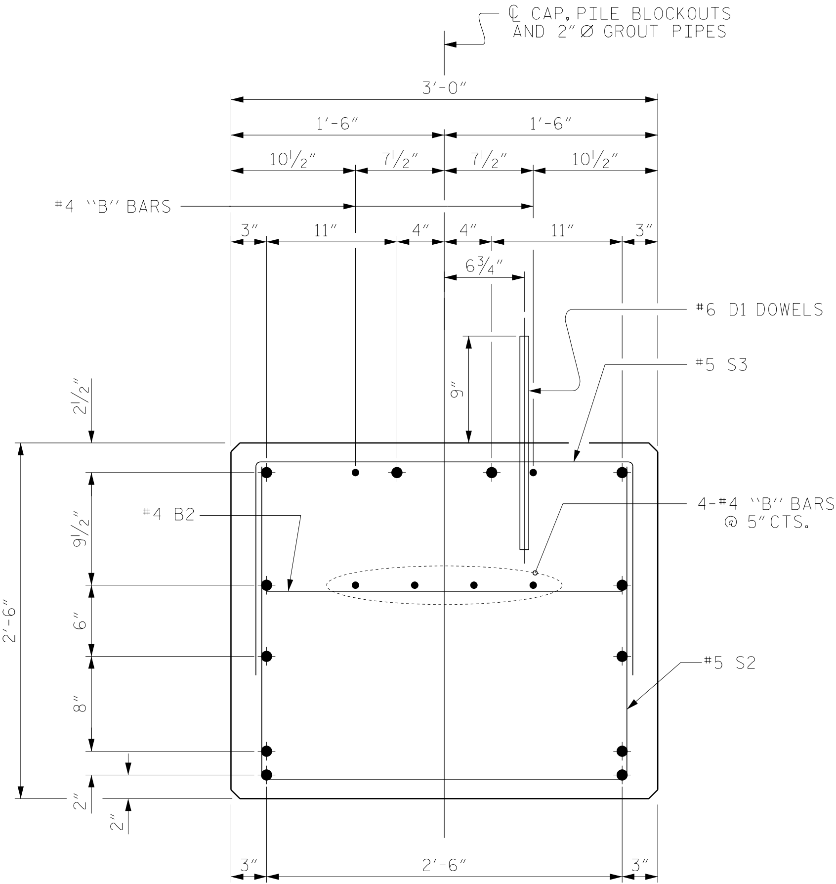
SECTION A-A
