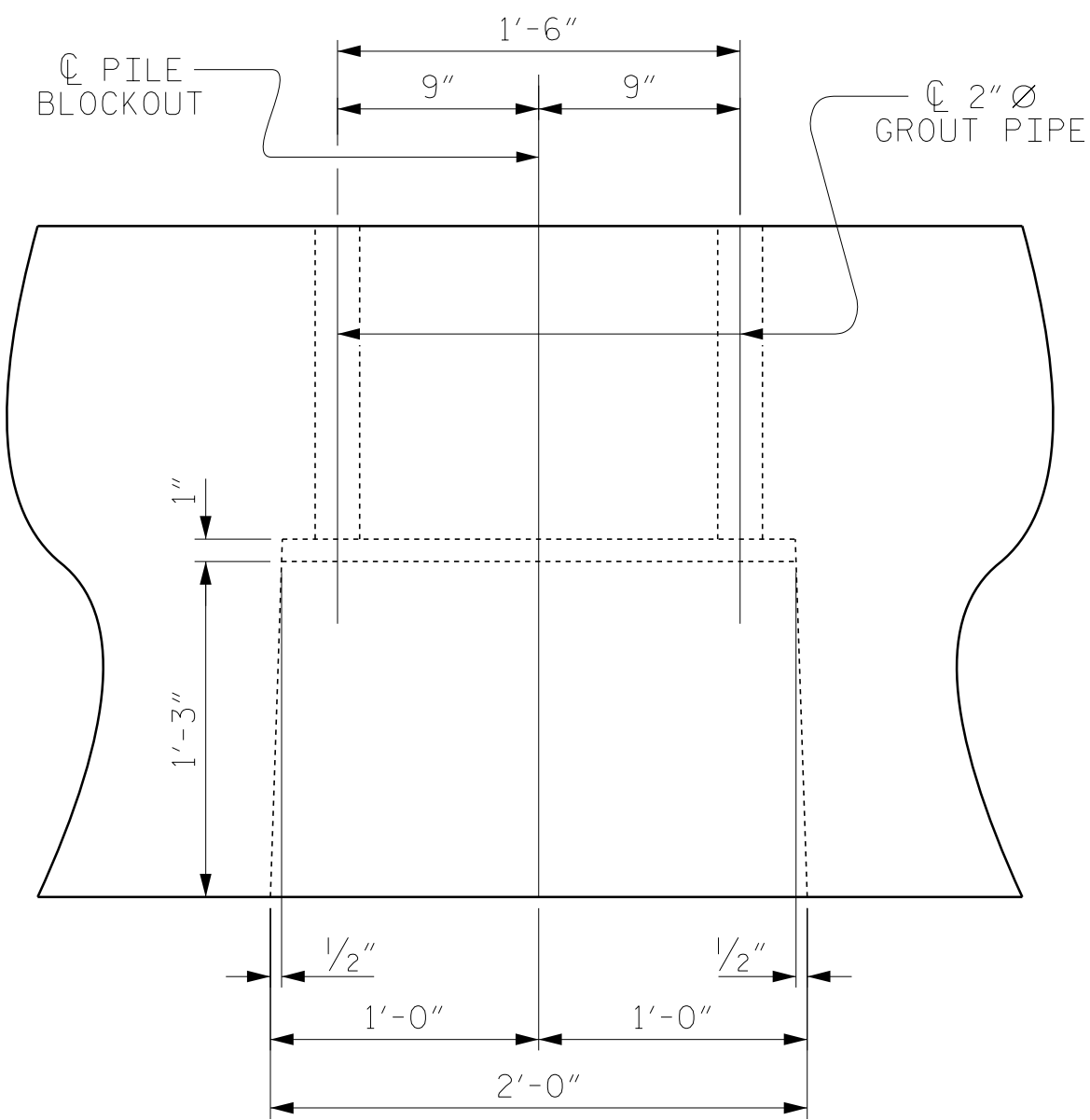
ELEVATION
