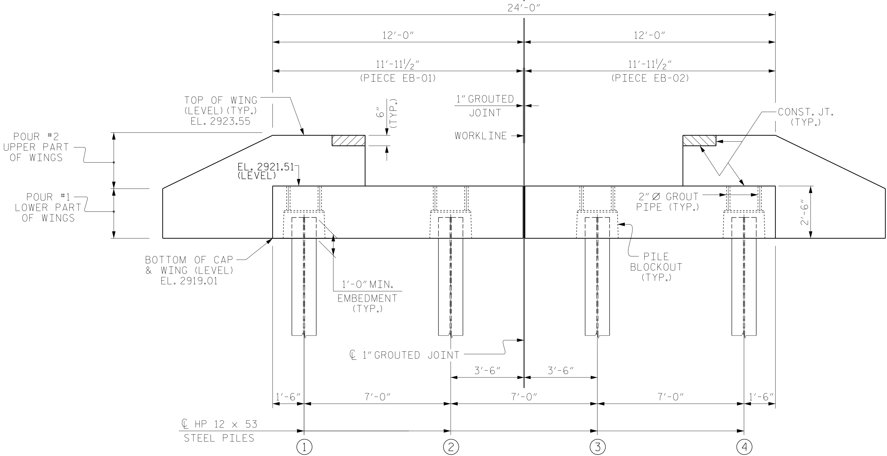
ELEVATION
