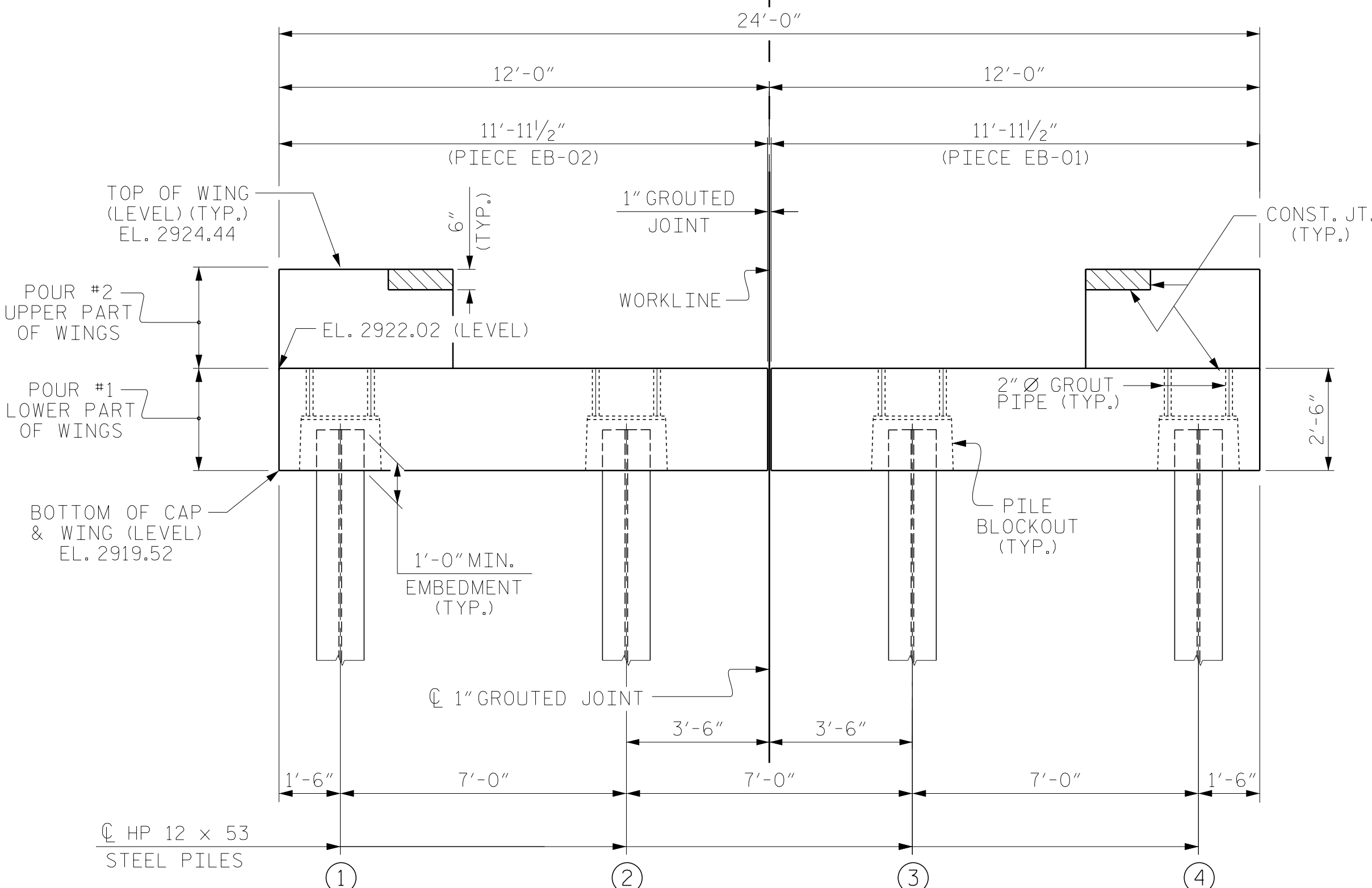
ELEVATION
